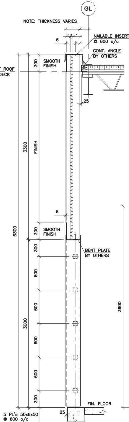
SECTION 2 TRUCK DOOR
